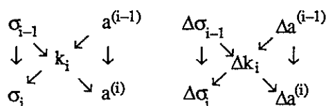
Figure 1. — Graphe de dépendance des variables calculées dans l'algorithme de LD.
